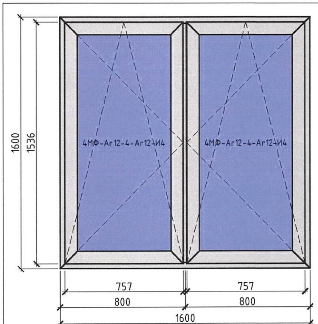
Рисунок 2—Схема образца 994-24-3. Взгляд со стороны помещения
